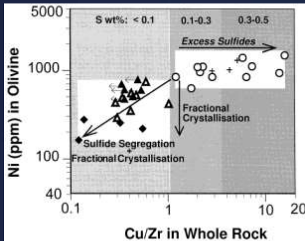
Figure présentant la composition d'olivines situées à proximité du gisement de Voisey's Bay (Li et Naldrett 1999)
